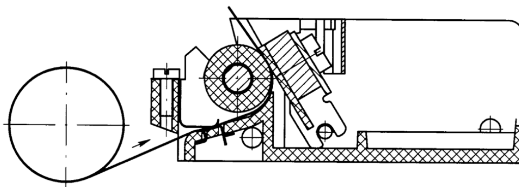
Рисунок 1 Схема заправки чековой ленты в ТПУ
